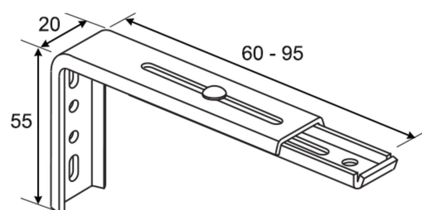
Équerre réglable 6-9.5cm
