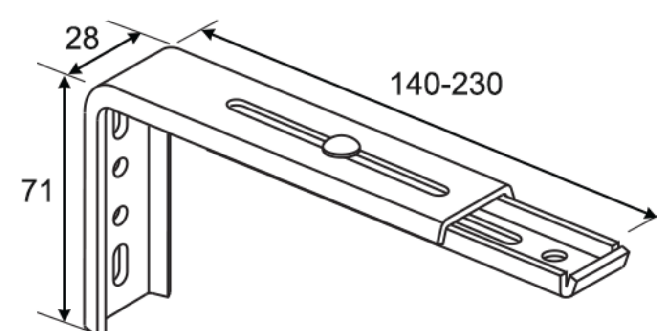
Équerre renforcée réglable 14-23cm
