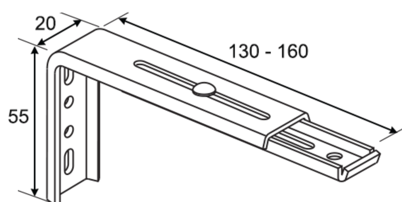
Équerre réglable 13-16cm
